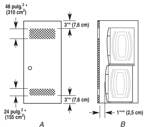
A. Aberturas de ventilación mínimas de las puertas del clóset B. Vista lateral de la lavadora y la secadora apiladas
